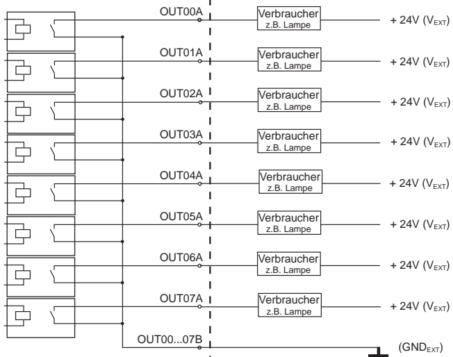
Prinzipschaltbild (gemeinsames GND)
