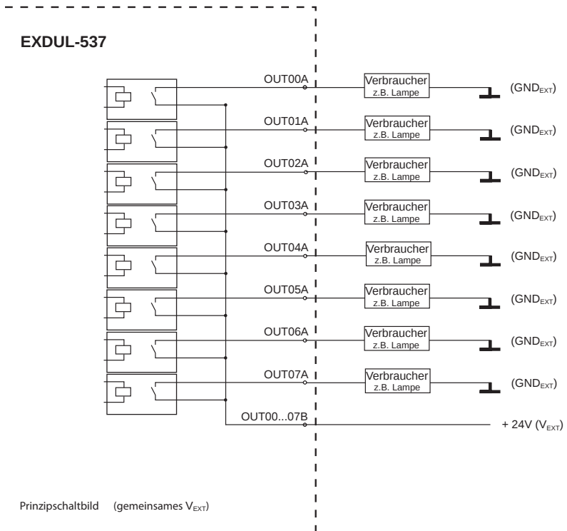
Grafik 17.2.2 Beschaltung der Optokoppler-Ausgänge revers
