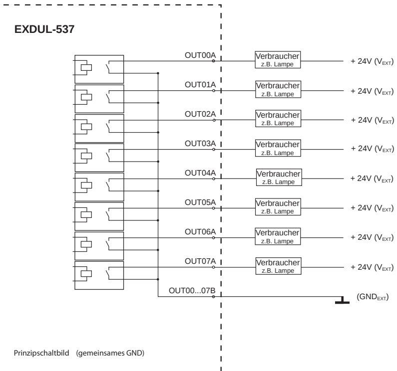
Grafik 17.2.1 Beschaltung der Optokoppler-Ausgänge
