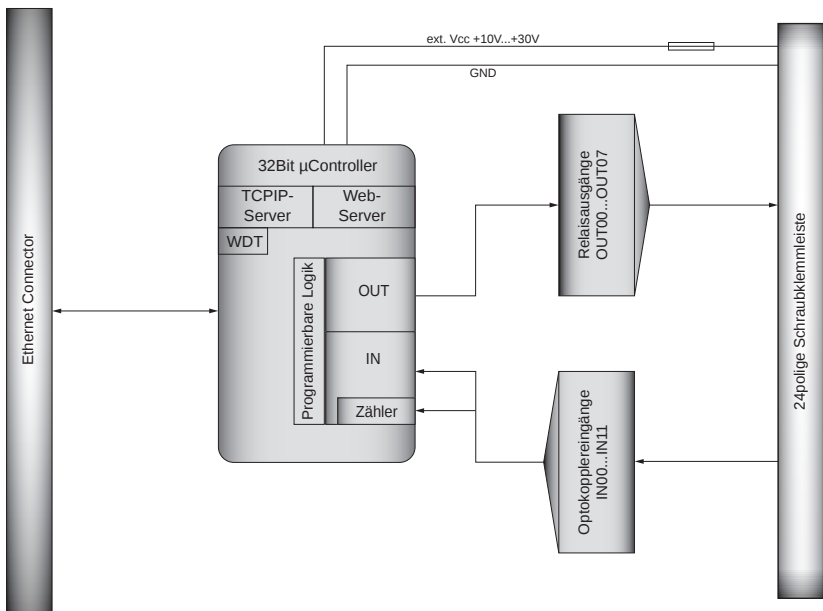
Grafik 3.3 Blockschaltbild EXDUL-537S
