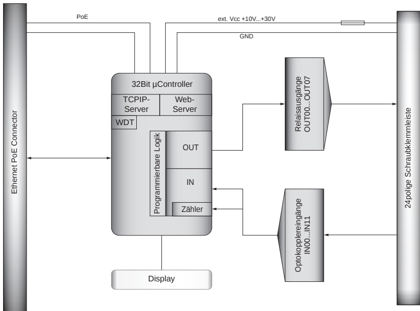
Grafik 3.1 Blockschaftbild EXDUL-537PoE
