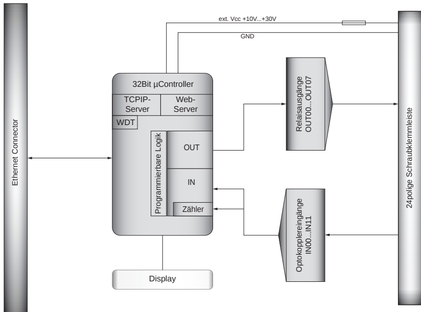
Grafik 3.2 Blockschaftbild EXDUL-537E
