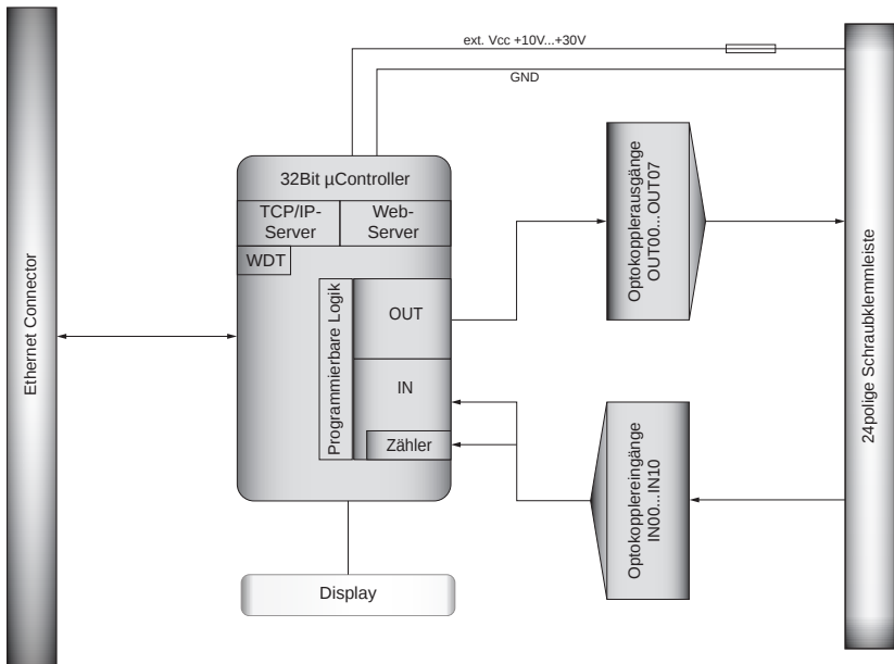
Grafik 3.2 Blockschaftbild EXDUL-519E
