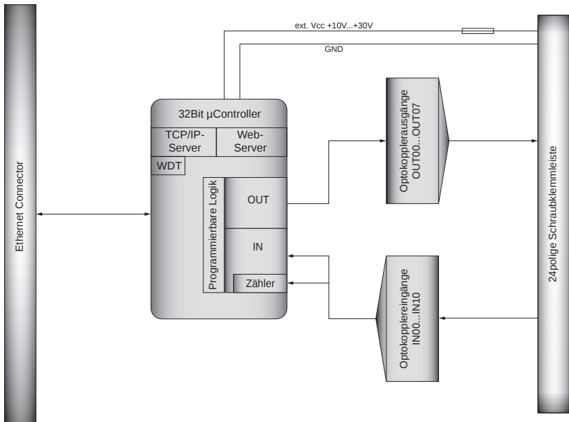
Grafik 3.3 Blockschaltbild EXDUL-519S
