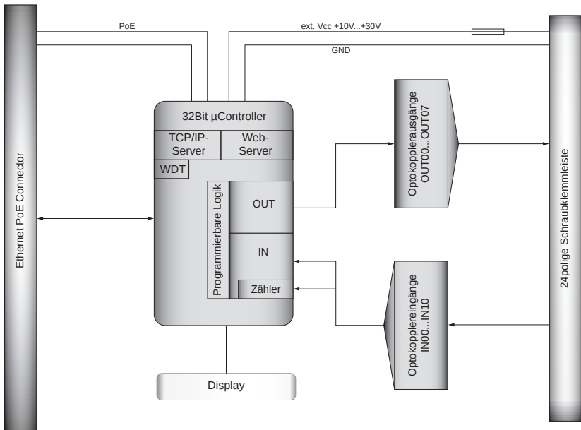
Grafik 3.1 Blockschaftbild EXDUL-519PoE
