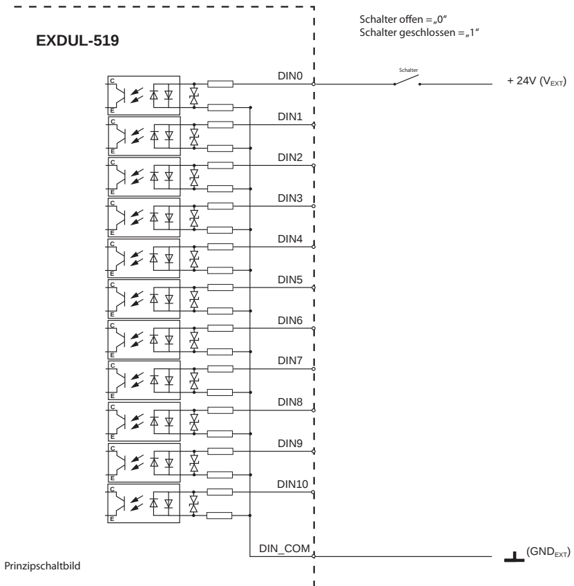
Grafik 17.1.1 Beschaltung der Optokopplereingänge
