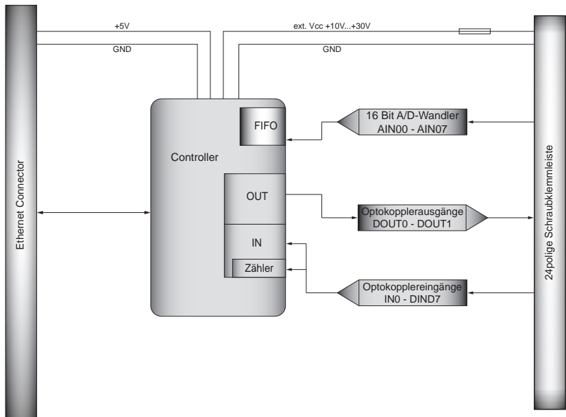
Grafik 3.3 Blockschaltbild EXDUL-581S
