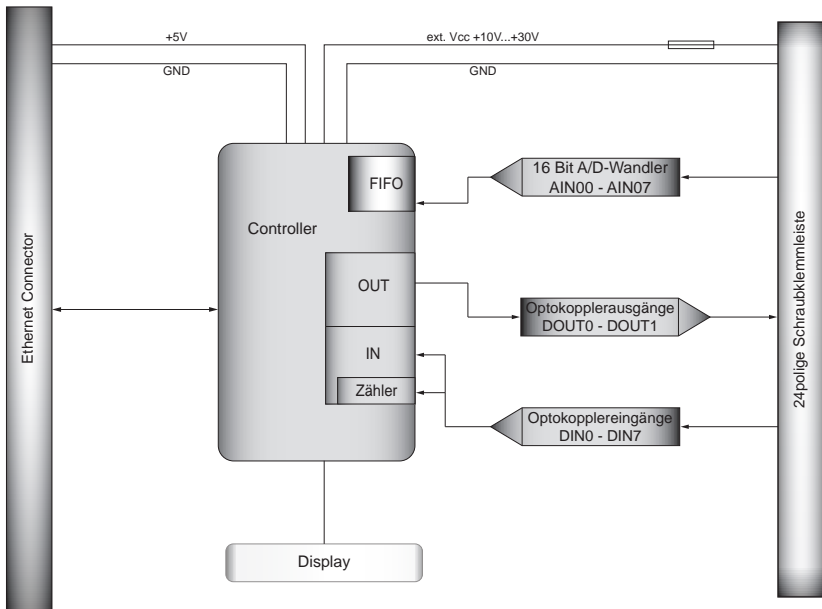
Grafik 3.2 Blockschahtbild EXDUL-581E
