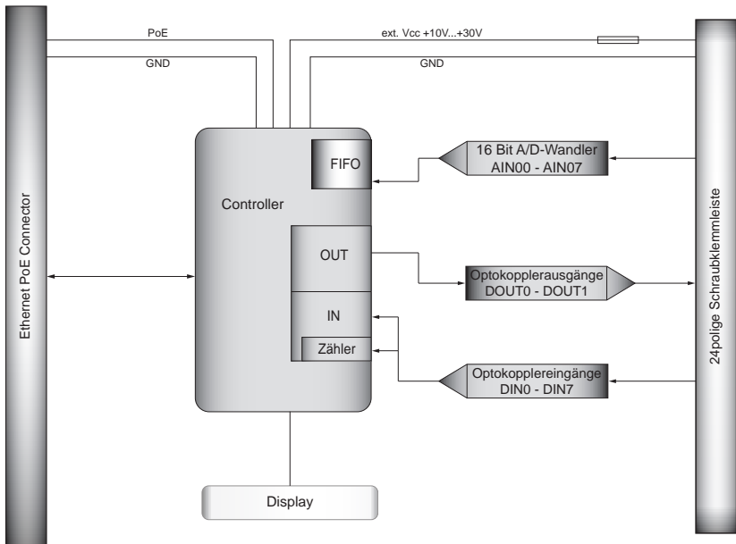
Grafik 3.1 Blockschahtbild EXDUL-581PoE
