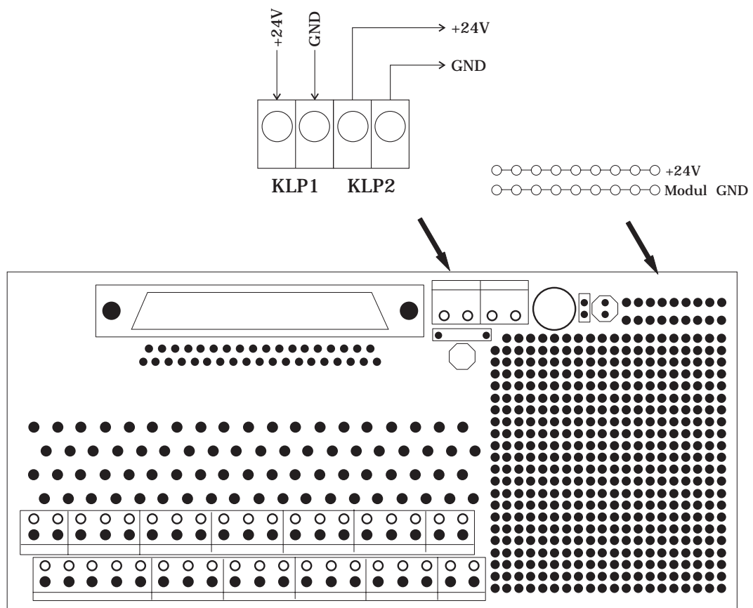
V+ und GND-Anschluß für Lochrasterfeld
