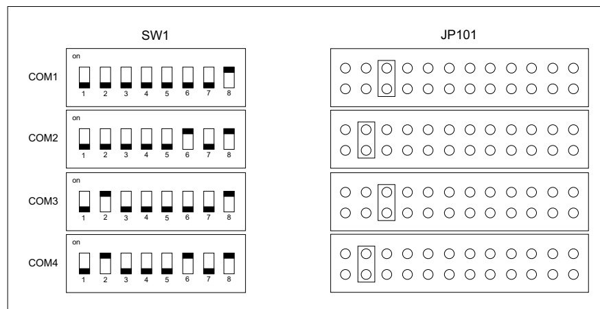
Schalter- und Jumperstellungen für COM1..COM4
