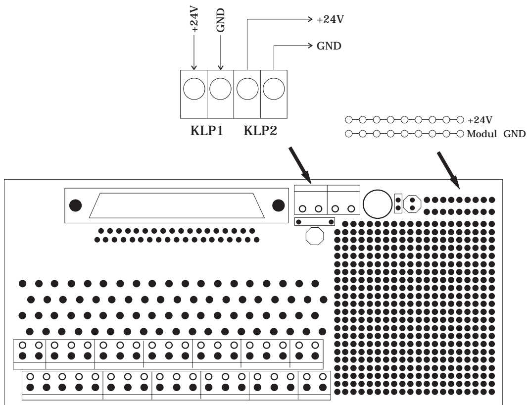
V+ und GND-Anschluß für Lochrasterfeld
