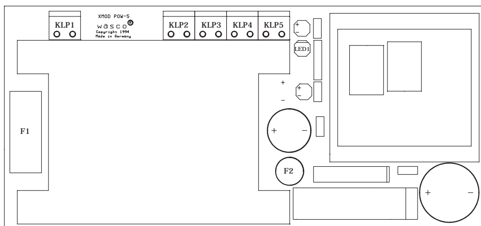
Abb.1-1 Komponentenlayout
