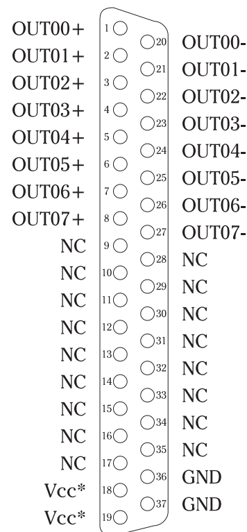
Abb.3-6 D-Sub-Buchse CND2
