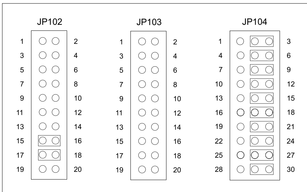
Jumpereinstellungen RS422 Modus
