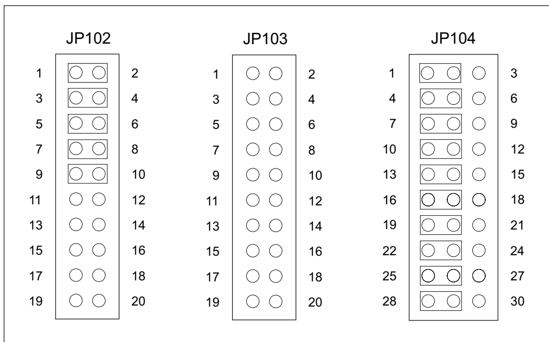
Jumpereinstellungen RS232 Modus
