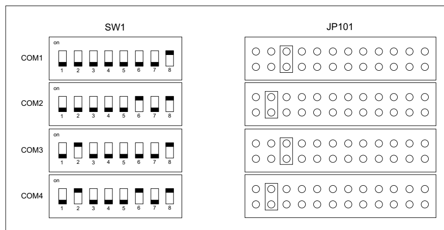
Schalter- und Jumperstellungen für COM1..COM4
